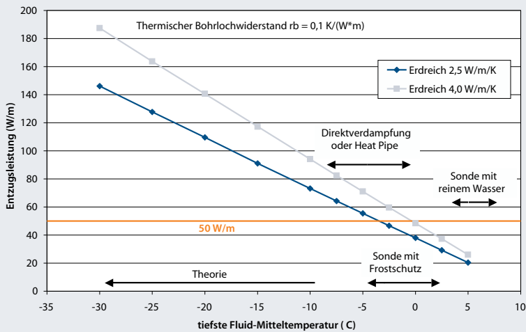
Abb. 9 Theoretisch mögliche Entzugsleistung für eine Erdwärmesonden-Anlage im Einfamilienhaus, 10 kW Heizleistung bei 1.800 Betriebsstunden im Jahr, berechnet für eine Sonde, gegen die tiefste Fluid-Mitteltemperatur aufgezeichnet; die Faustformel 50 W/m und typische Bereiche für Erdwärmesonden-Bauarten sind angegeben.
